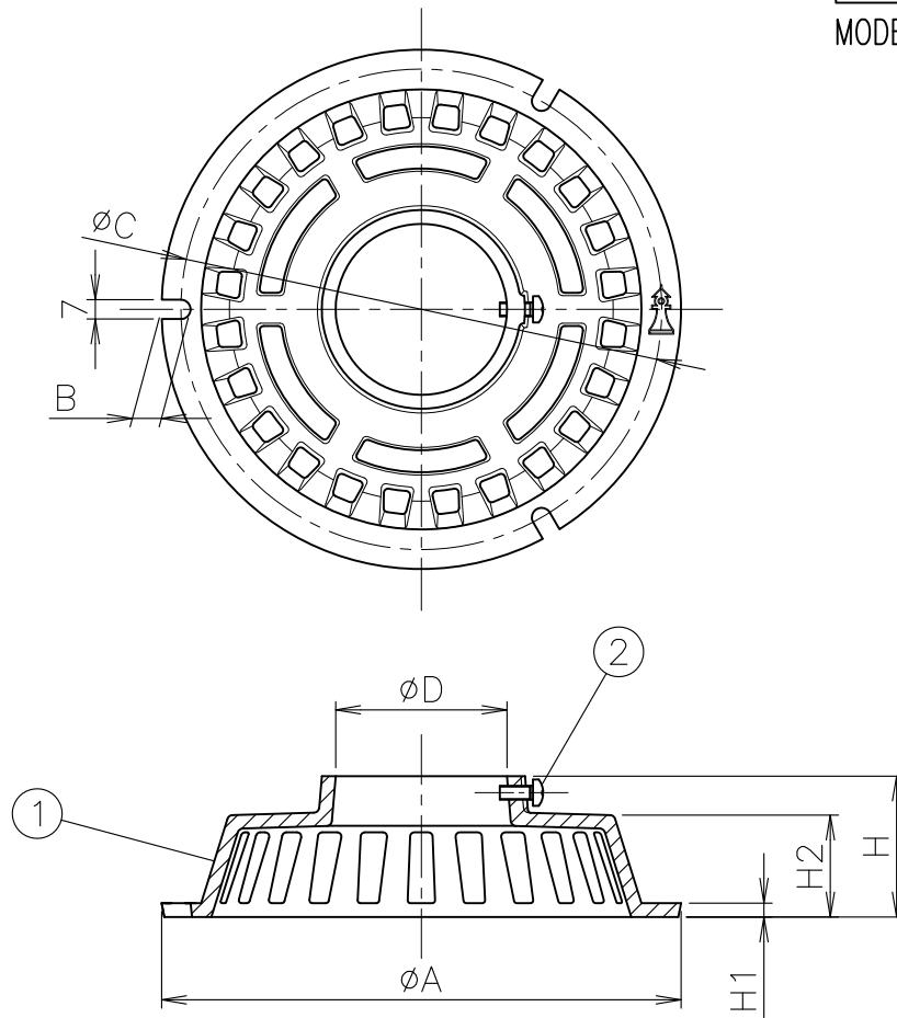
寸法表
